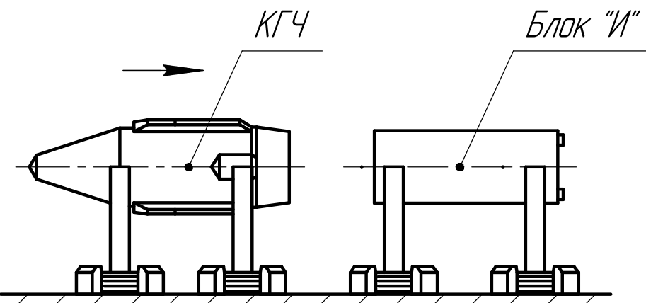
5.2. Стыковка КГЧ с блоком "И"
