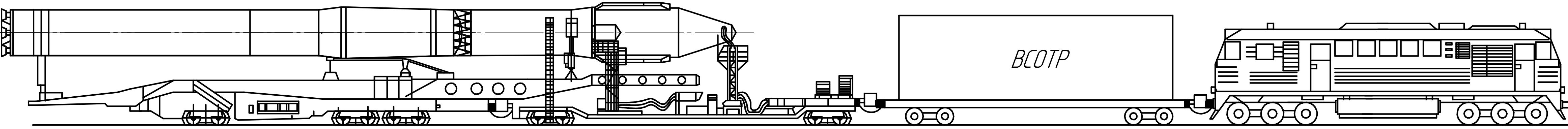
8. Транспортировка РКН Союз-2.1в на стартовый комплекс
